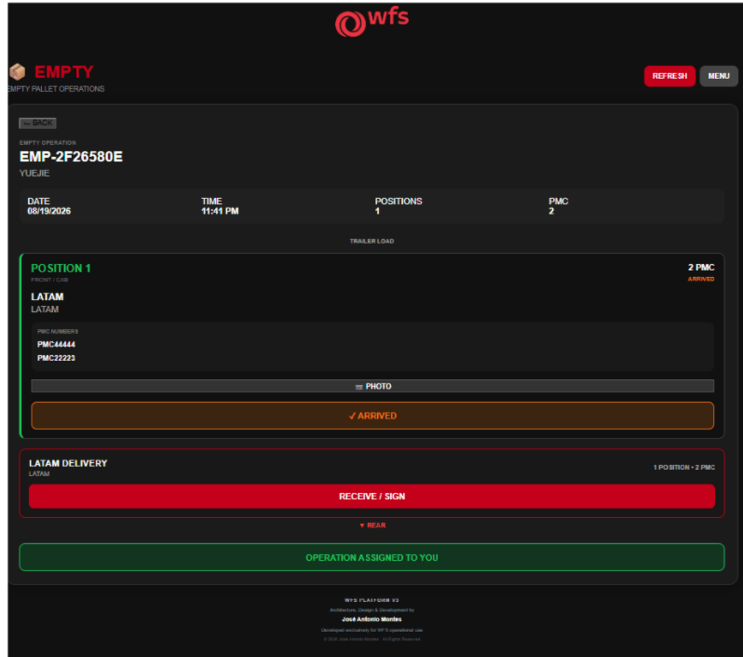
Captura del módulo desarrollado en WFS Platform V3
